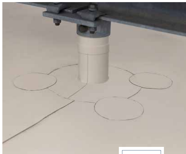
Die 260 individuell angefertigten Stützeneinfassungen für die PV-Aufständerungen erleichterten die Abdichtungsarbeiten maßgeblich
