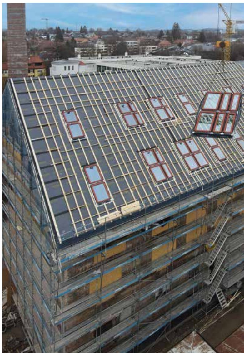
Einbau der vormontierten Dachfensterelemente
